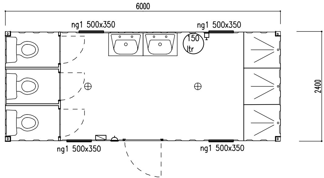
PLAN 1:50
