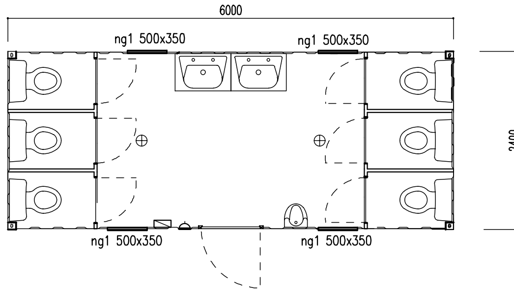
PLAN 1:50
