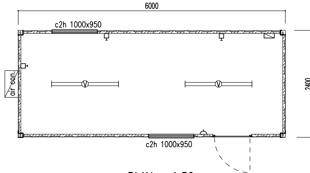
PLAN. 1:50
