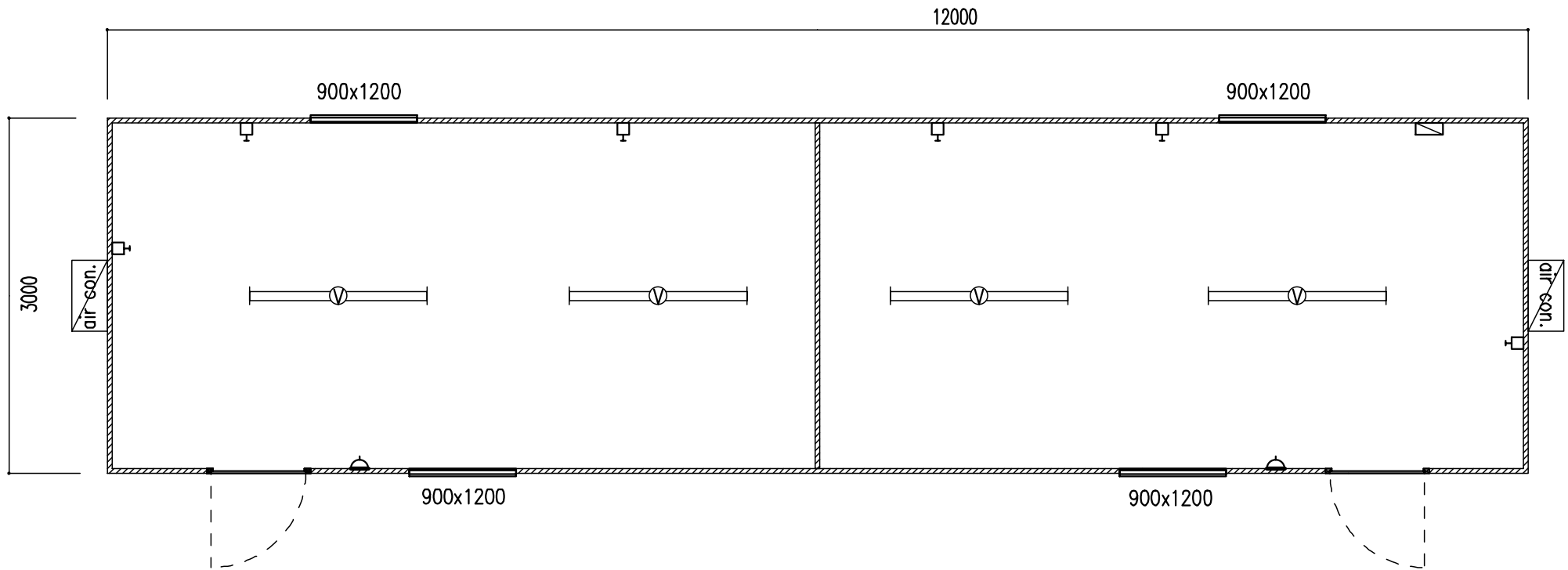
PLAN. 1:50
