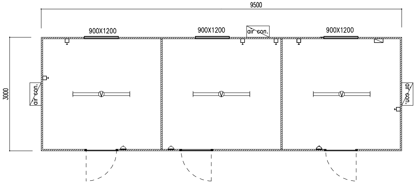
PLAN. 1:50
